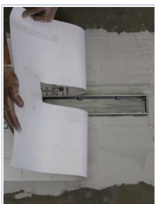
21 exemplo de aplicação do centro de impermeabilização LINEA CONFORT e COMPACT mantendo-se todos os passos de 1 a 19
