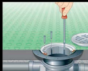
O revestimento é fixado ao ralo de pavimento com a flange aparafusada
