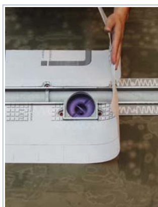
22 exemplo de aplicação do centro de impermeabilização LINEA SUPER G 60 mantendo-se todos os passos de 1 a 19
