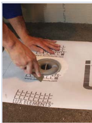
7 aplique o centro de impermeabilização sobre a flange e apertar com ajuda de uma espátula
