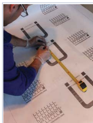
7 marcar o centro da lâmina para retirar o quadrado de sobreposição no centro.
