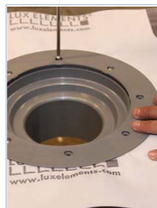
20 exemplo da aplicação do centro de impermeabilização série PERFECT mantendo-se todos os passos anteriores
