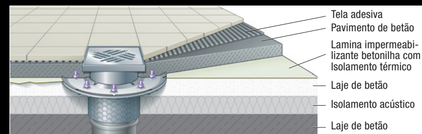
Vedação através de membrana isolante e flange de compressão.
