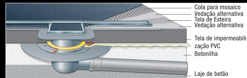
Vedação convencional usando tela de isolamento
