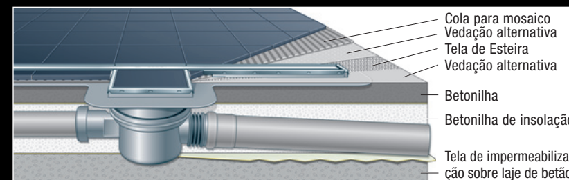
Impermeabilização executada sobre a flange do canal
