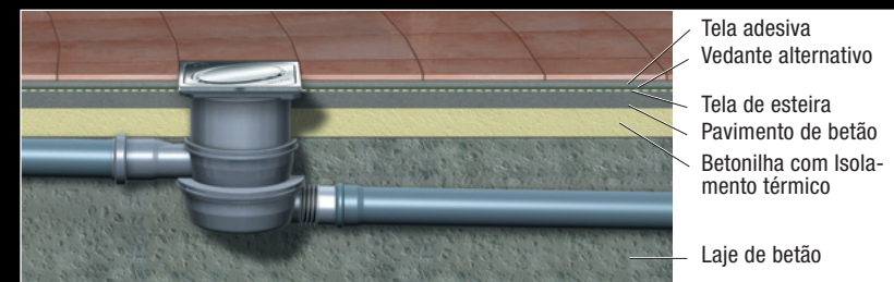
Ralo com flange superior para conexão de vedante alternativo
